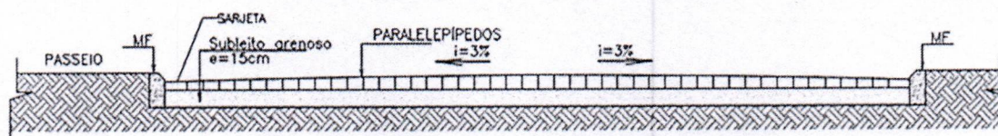
Figura 1 - Seção transversal.
