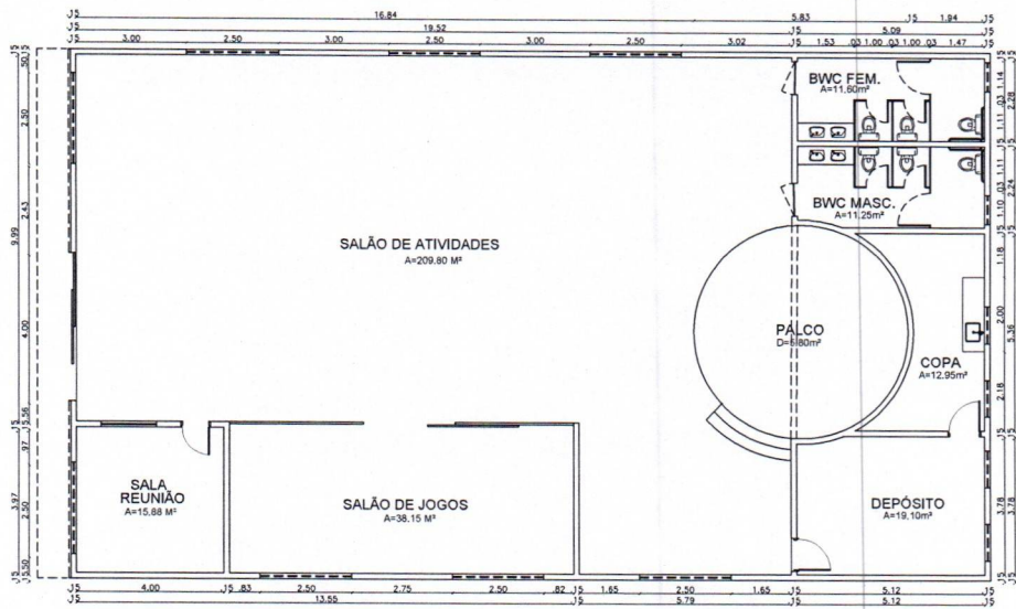
PLANTA BAIXA ESCALA _____ 1/100
